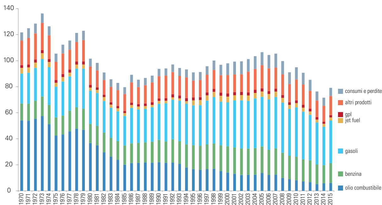
Italia - Evoluzione della produzione delle raffinerie (Milioni di tonnellate)
