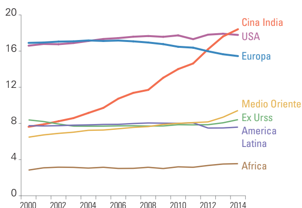
Mondo - Capacità di raffinazione per area geografica (Milioni di barili/giorno)
