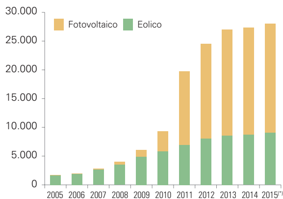
Italia - Potenza installata da fonti energetiche rinnovabili non programmabili (GW)
